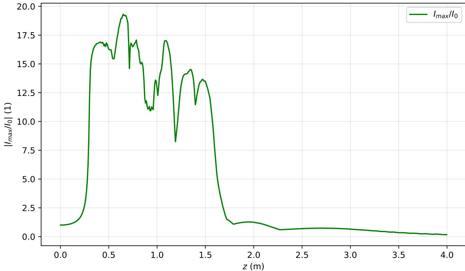
I_{\max}(r=0, z)/I_0 , Pin=9.3Pcr
